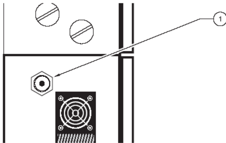
图 2-36 排气口连接
